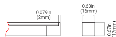
End Cap #052286
