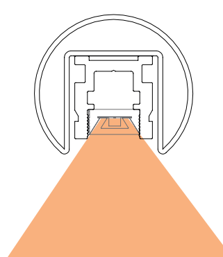
1.6" OD Handrail
